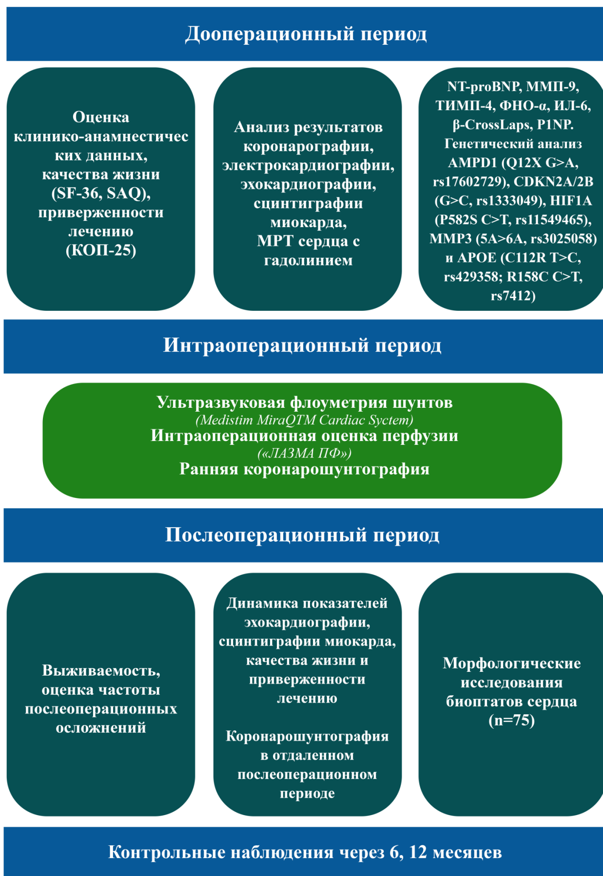
Рисунок 1. Методы исследования
